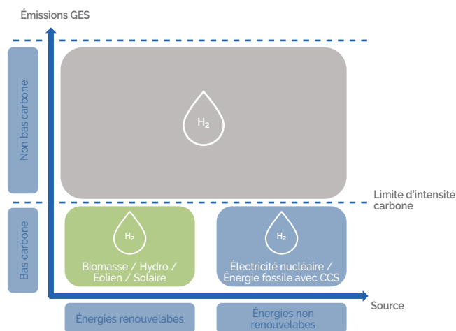
Classification de l'hydrogène par modes de production développée dans le cadre du projet CertifHy 25
